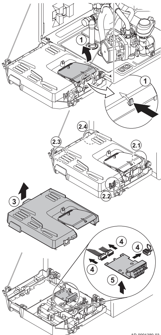
Afb.220 Toegang tot de aansluitconnectoren
