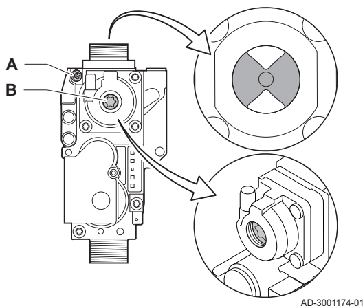
Afb.68 Gasblok
