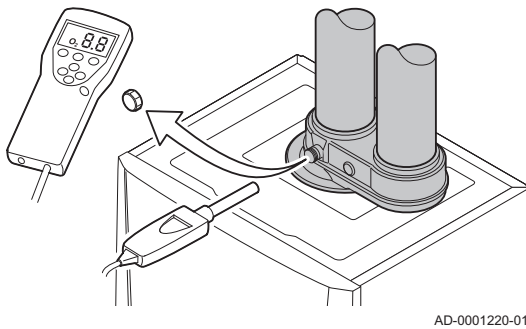
Afb.61 Rookgasmeetpunt
