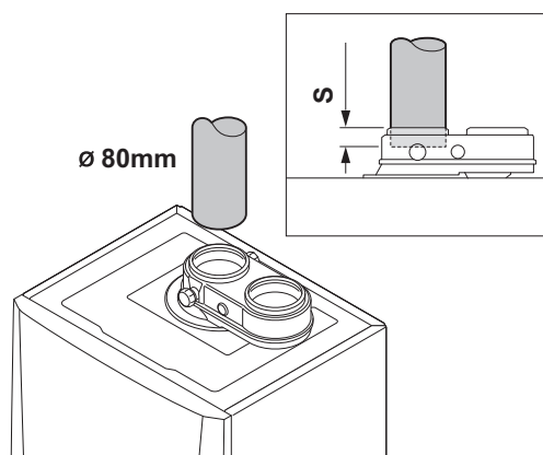
Afb.40 Aansluiten rookgasafvoer (parallel)
