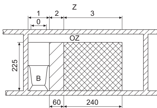
Afb.16 Badkameropstelling
