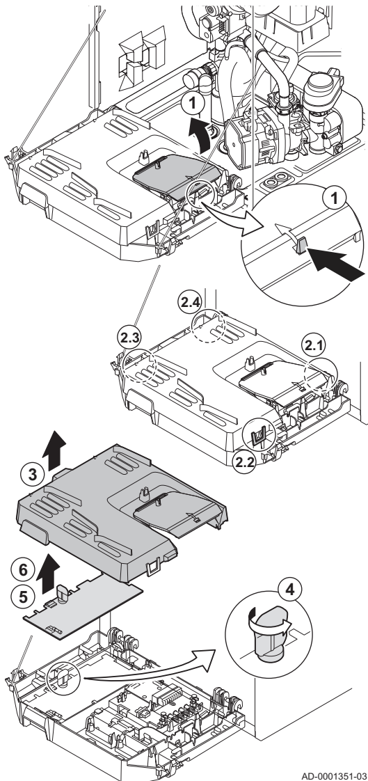
Afb.219 Toegang tot de aansluitconnectoren
