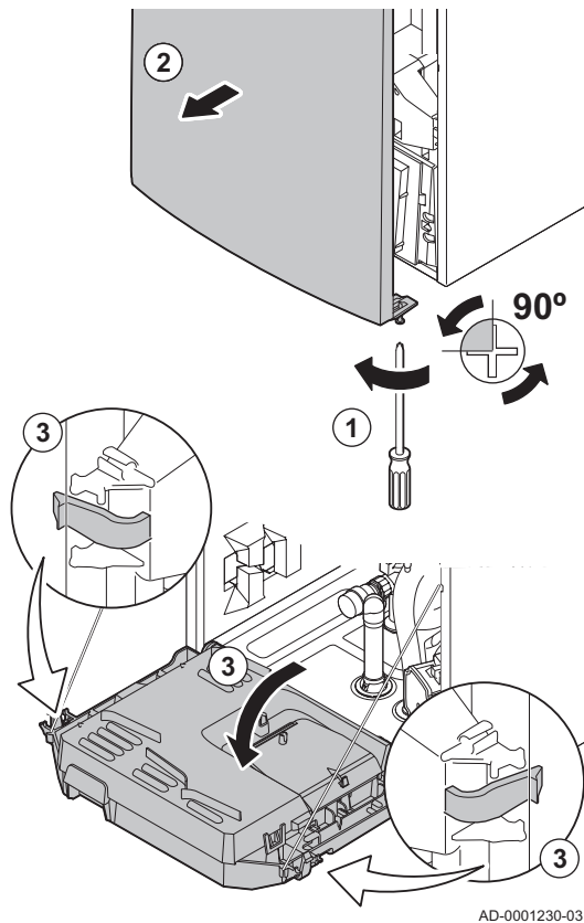
Afb.212 Ketel openen
