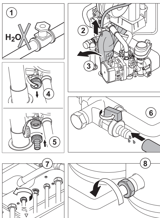
Afb.216 Vervangen boilervaten
