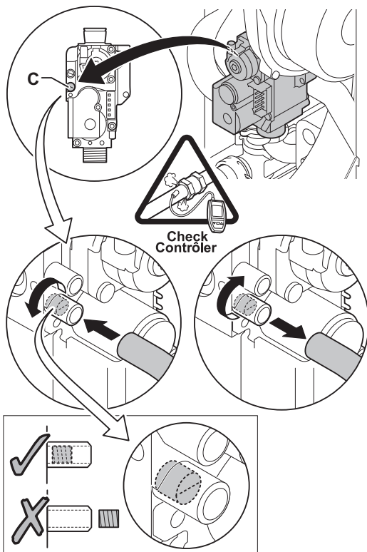
Afb.60 Gasblok meetpunten
