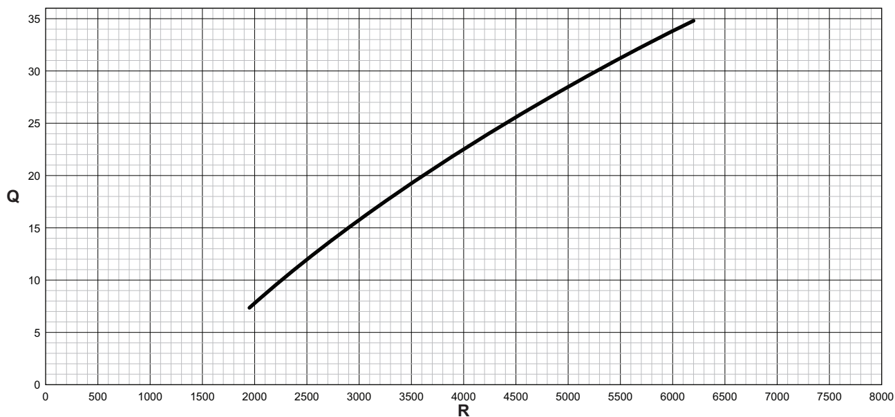
Afb.201 Grafiek voor Calenta Ace 40L
