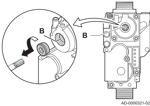
Afb.67 Positie afstelschroef B
