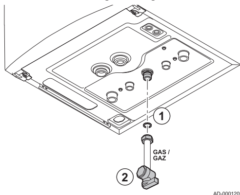
Afb.25 Aansluiten gasleiding
