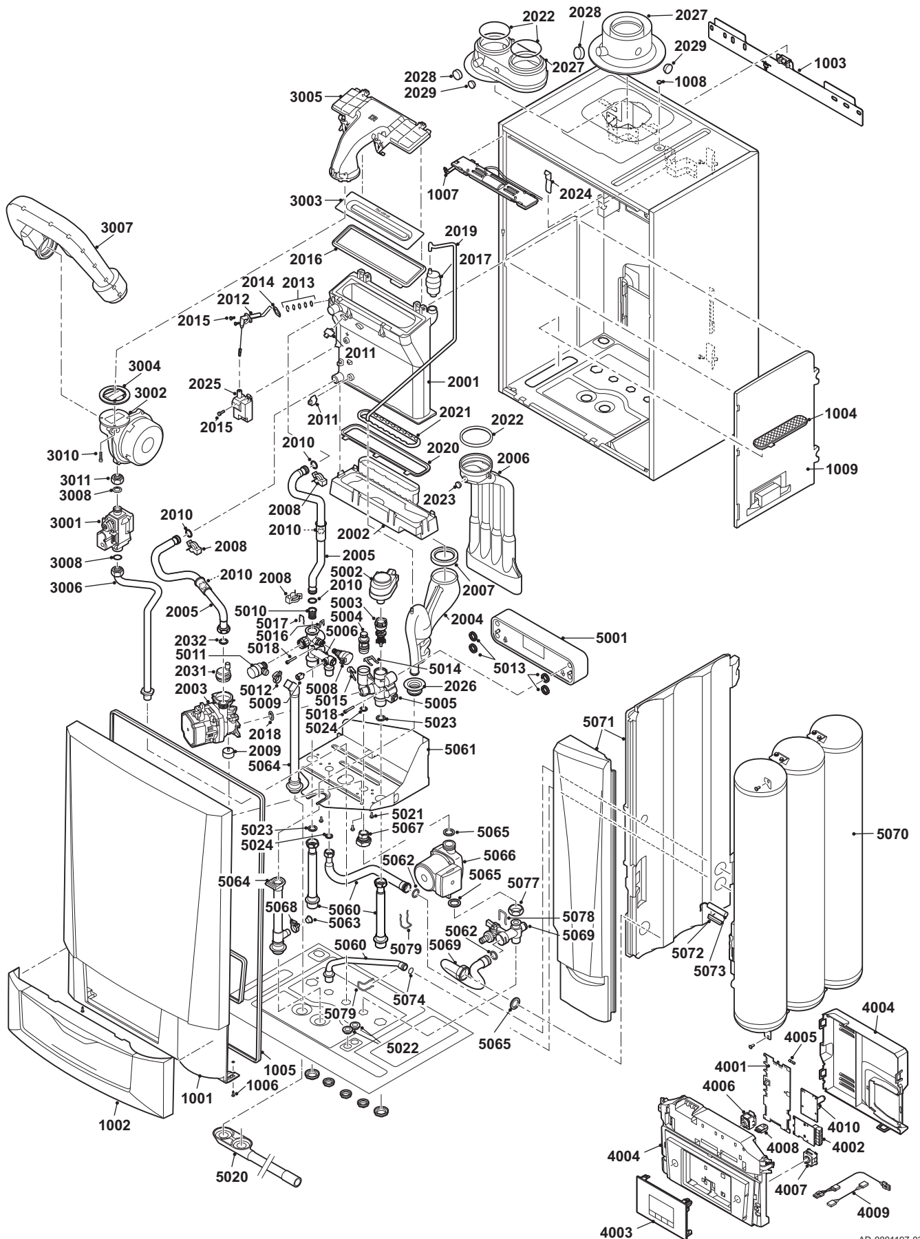
Afb.247 Calenta Ace 40L
