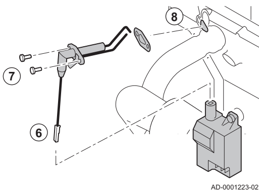
Afb.213 Vervanging van de ionisatie-/ontstekingselektrode
