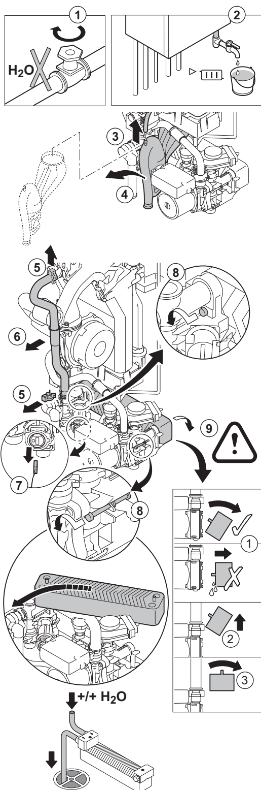
Afb.214 Reiniging platenwarmtewisselaar
